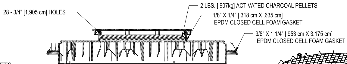
SECTION A-A
